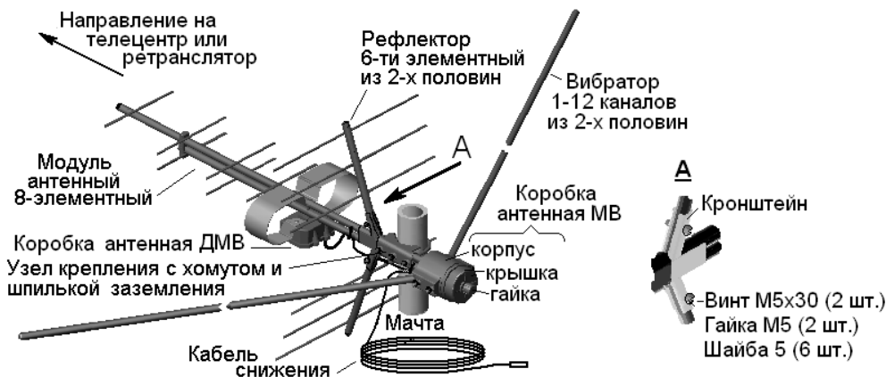
Рисунок 1 - Сборка и установка антенн на месте эксплуатации
