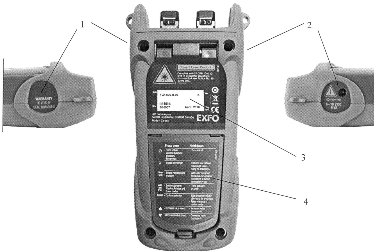
Рисунок 2 - Схема корпуса тестера – вид сзади/сбоку
