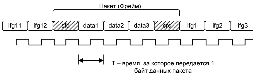
Рисунок 20-2. Передача фреймов и тактовый сигнал.
