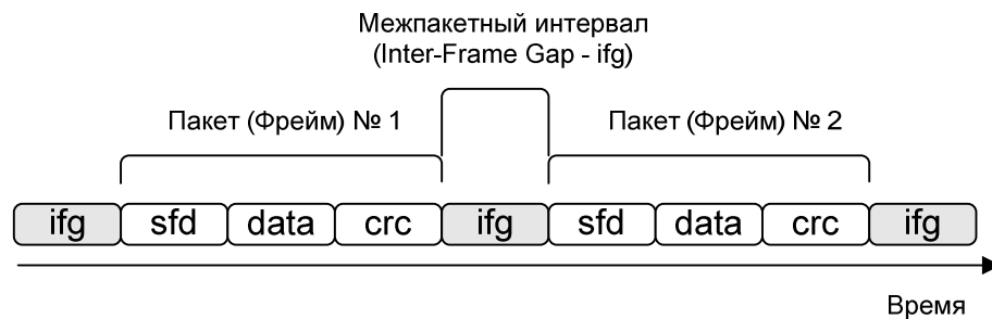
Рисунок 20-1. Передача фреймов
