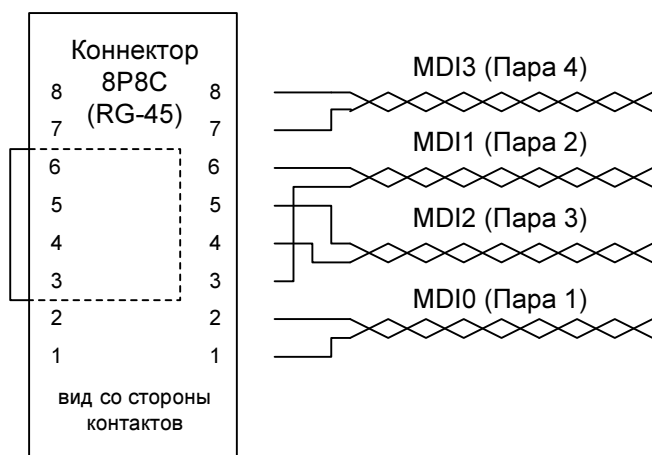
Рисунок 17-2. Правильное подключение.
